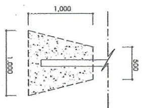
기조 상세도 S=1:20
